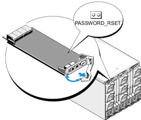
Abbildung 12-1. Kennwort-Reset-Jumperposition
