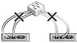
Abbildung 2-2. Inkorrekte Verkabelung für CMC-Netzwerkverbindung - 2 CMCs
