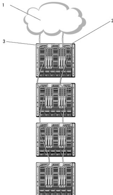
Abbildung 2-1. Verkettete CMC-Netzwerkverbindung
