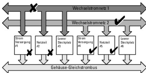
Abbildung 9-1. Abbildung 8-2. 2 Netzteileneinheiten pro Netz und ein Stromausfall in Netz 1
